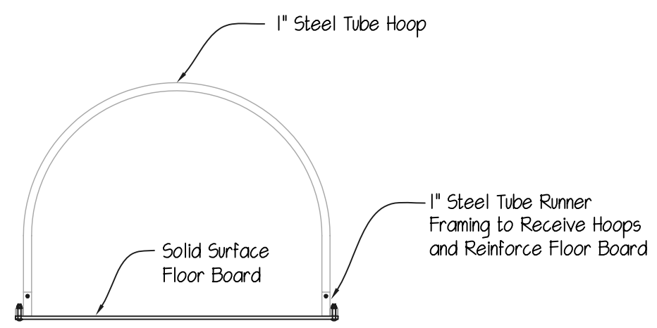
END ELEVATION
